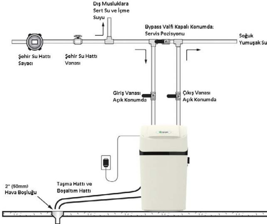
Şekil 12: Servis Pozisyonu
