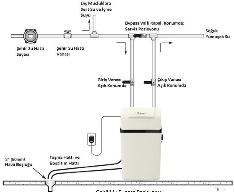
Şekil 11: Bypass Pozisyonu
