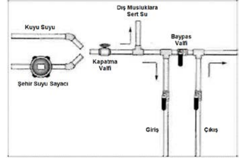
Şekil 6: Üç Yönlü Bypass Tesisatı
