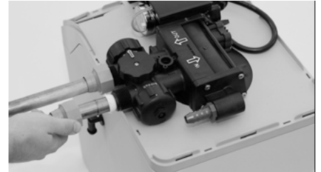
Şekil 8: Su Hatlarını Bağlayın (Bypass Valfi ile Gösterilmiştir)
