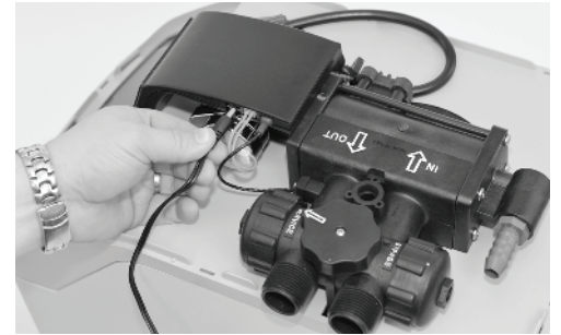
Şekil 15: Transformatör Güç Kablosunu Bağlayın
