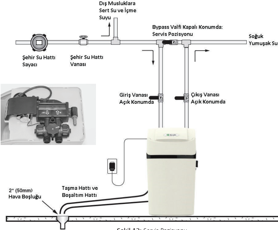
Şekil 13: Servis Pozisyonu
