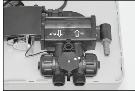
Şekil 17: Bypass Valfi
