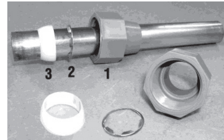
Şekil 8: Quest Bağlantı Elemanları
