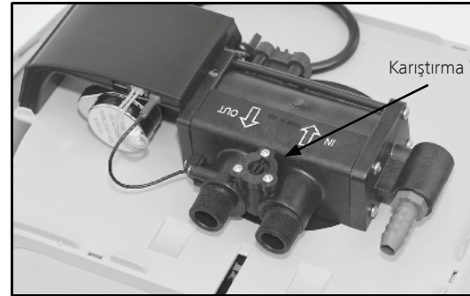
Şekil 18: Karıştırma Vanasının Ayarlanması
