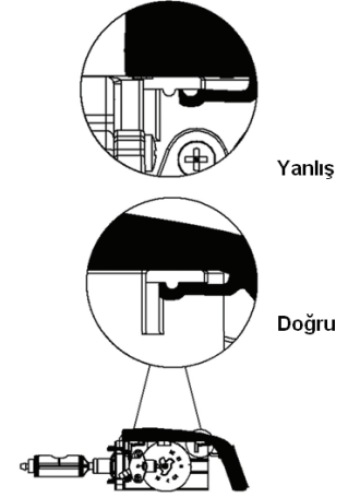
Şekil 14: Kontrol Cihazı Sekme Kilit Ayrıntısı
