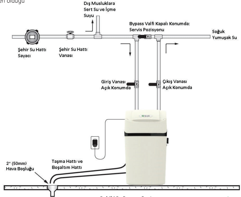
Şekil 12: Bypass Pozisyonu
